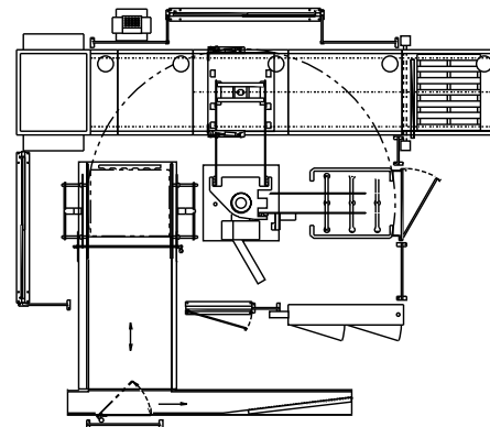
Paletizador/Despaletizador Completamente Automatico
