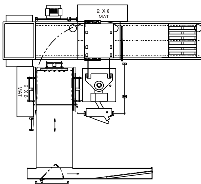
Paletizador/Despaletizador Semi-Automatico Con Manejo de Pallet Totalmente Automatico
