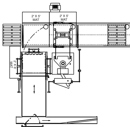
Paletizador/Despaletizador Semi-Automatico
